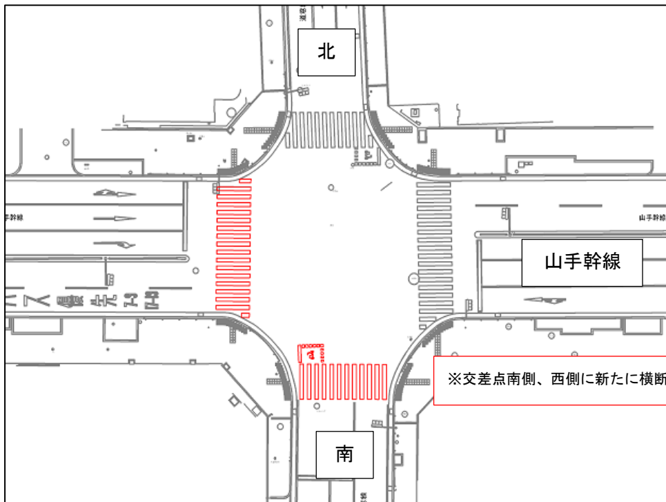
桂木交差点 改良平面図
