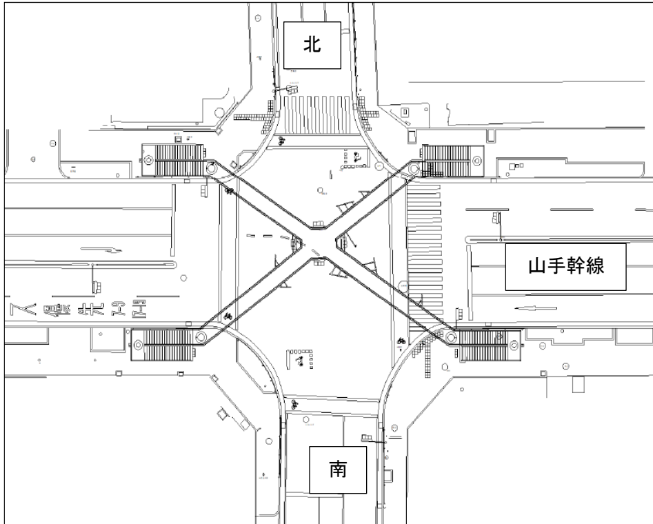
桂木交差点 現況平面図
