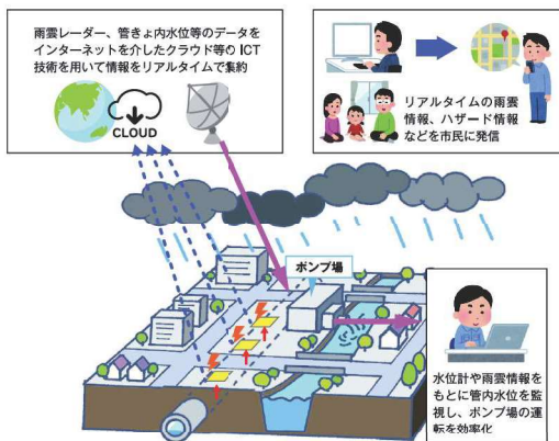
下水の流入予測技術の研究
