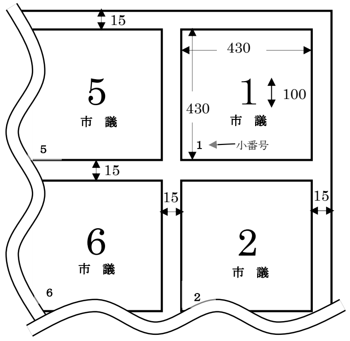
(野立設置例) 単位：ミリ
