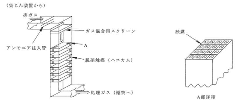
触媒脱硝反応塔
