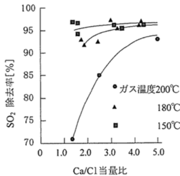
消石灰噴霧の場合の除去性能例（温度の影響）
