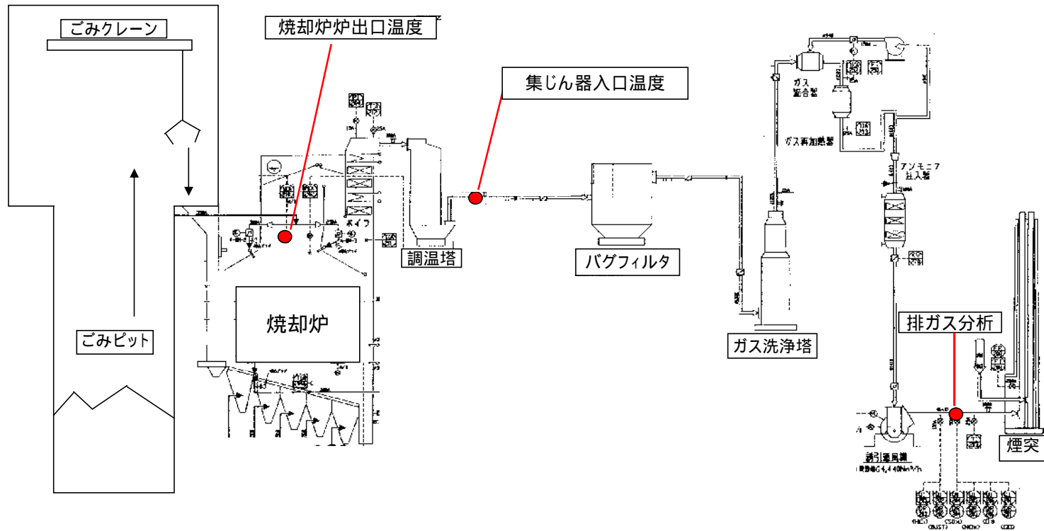
第1工場 処理工程概要図
