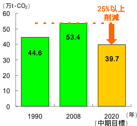
家庭部門の二酸化炭素排出量の推移と目標
