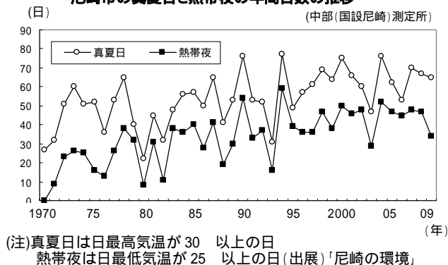
尼崎市の真夏日と熱帯夜の年間日数の推移
