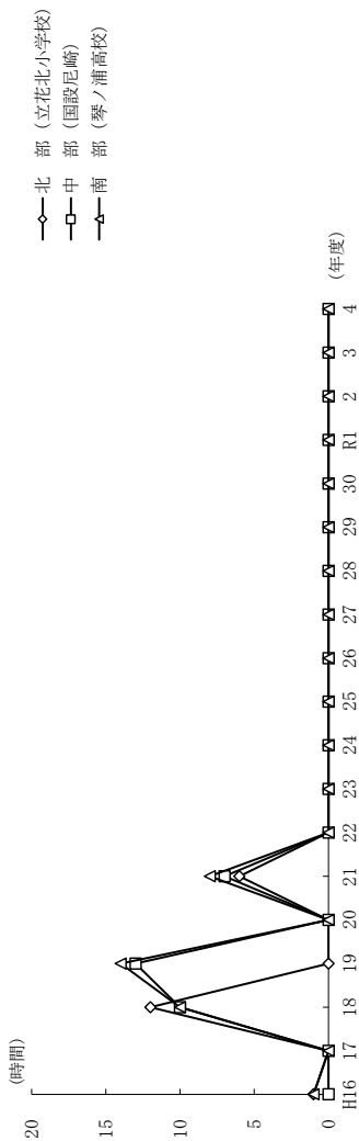
浮遊粒子状物質の推移（一般環境大気）1時間値が0.2mg/m 3 を超えた時間数
