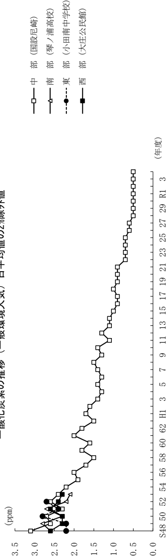
一酸化炭素の推移（一般環境大気）日平均値の2%除外値
