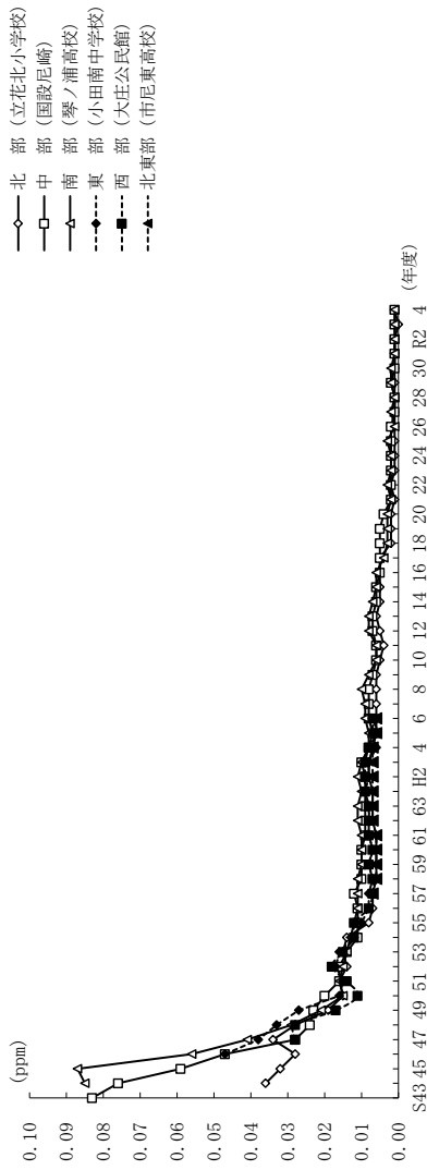
二酸化硫黄の推移（一般環境大気）年平均値
