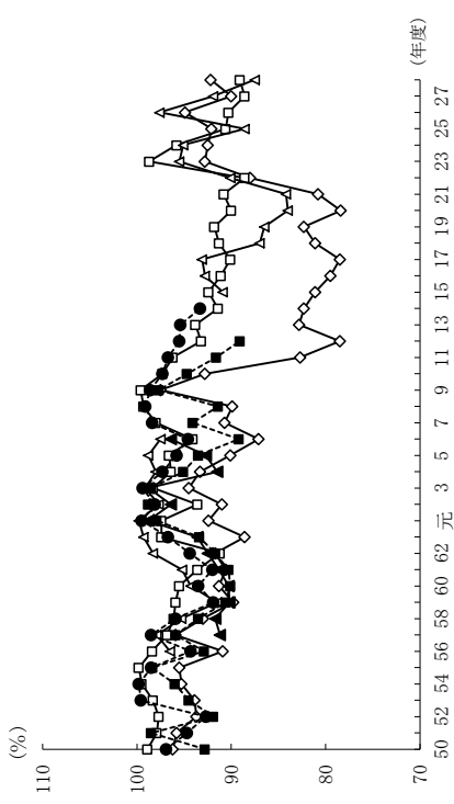
屋間オキシダント濃度の環境基準適合率の推移（一般環境大気）期間〔4月～10月〕時間適合率
