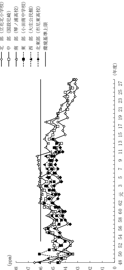
二酸化窒素の推移（一般環境大気）日平均値の年間98%値
